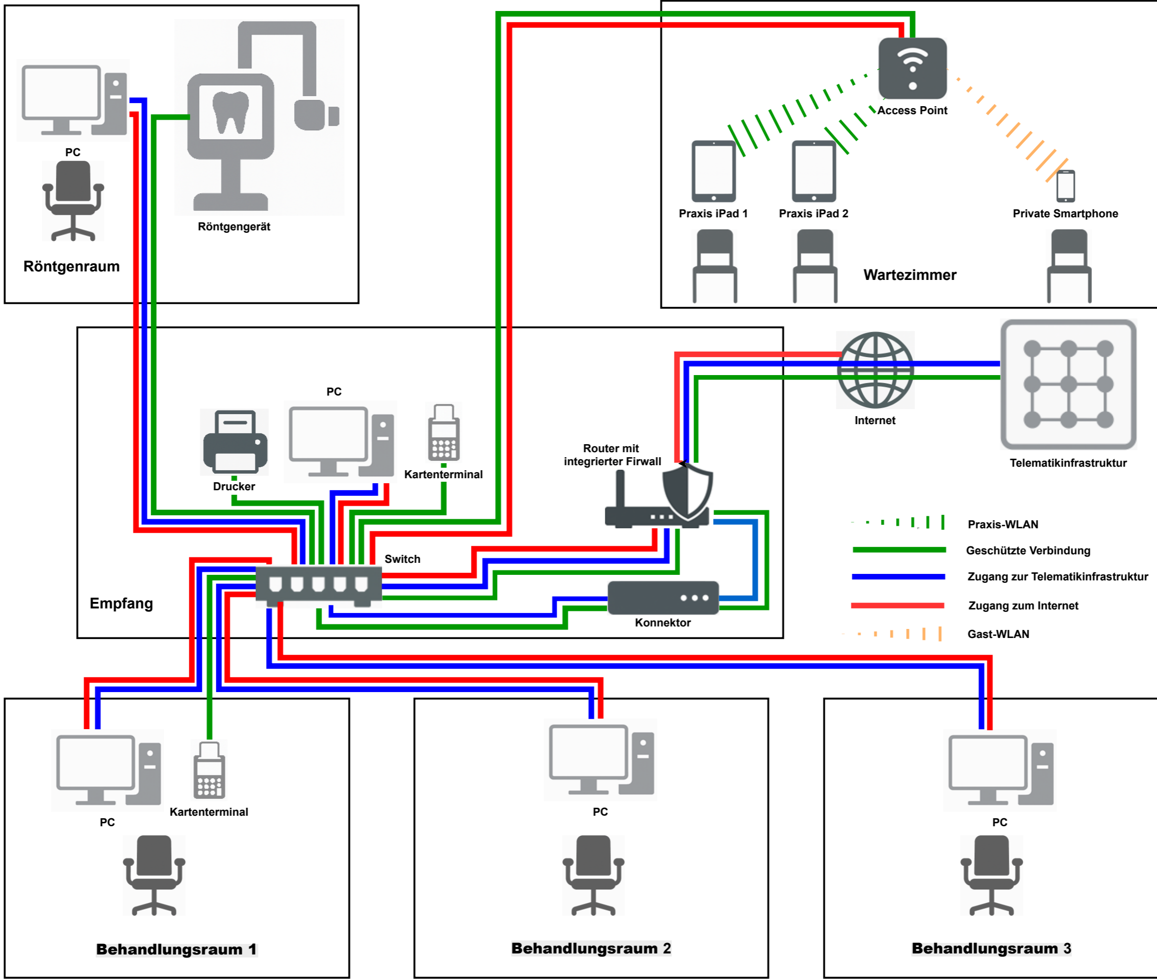
Abbildung: Beispiel-Netzplan einer Praxis mit Parallelbetrieb
